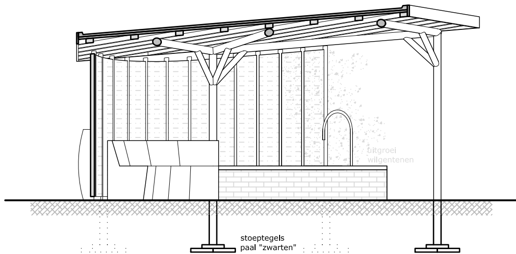
Doorsnede - 1:50
