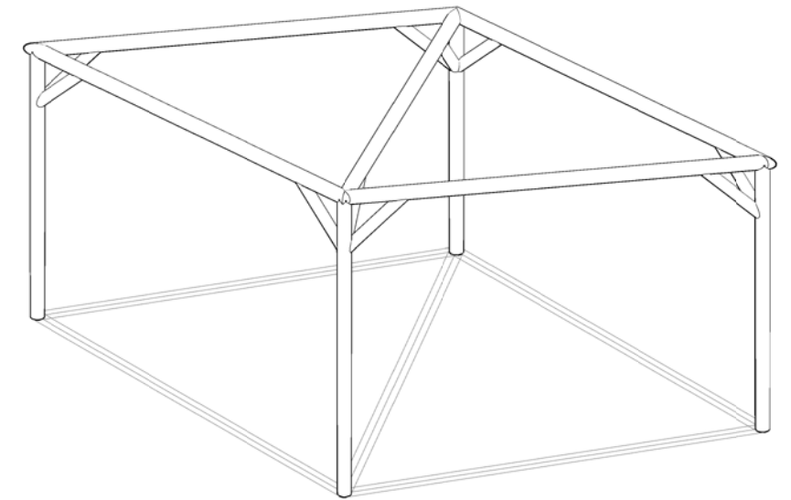
Isometrie hoofdconstructie
