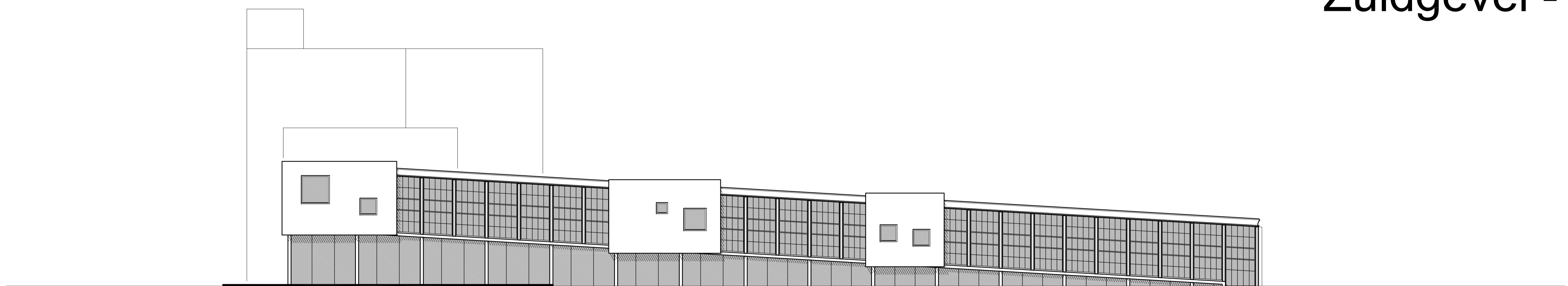
Oostgevel - 1:200
