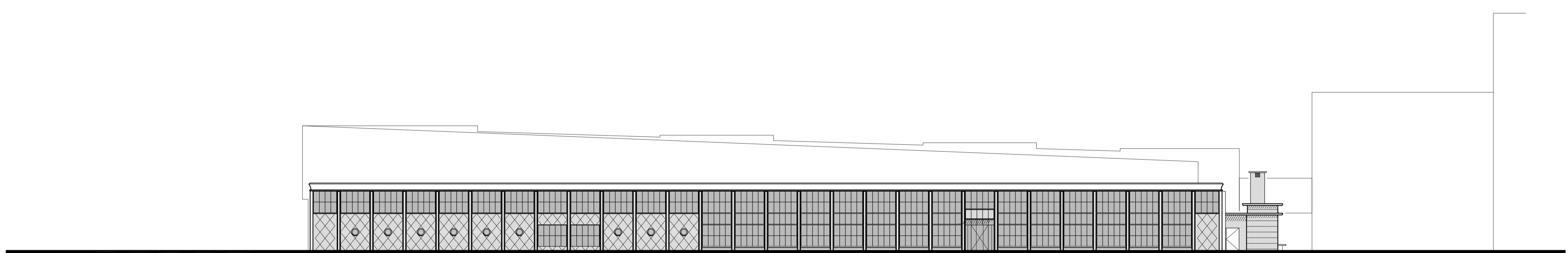
Noordgevel - 1:200
